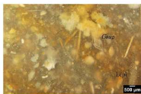
3 : texture wackestone à Spicules, Goupillaundina et Lépidodictya, échelle 500 µm.
